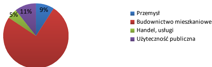
Rysunek 12. Struktura sprzedaży ciepła sieciowego w całkowitym zużyciu w poszczególnych grupach odbiorców w 2013 roku 120
