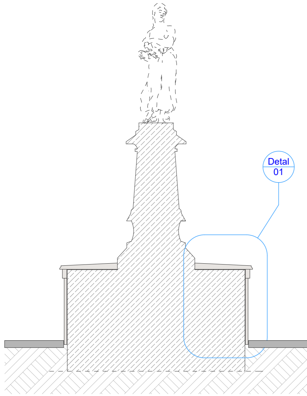
PRZEKRÓJ A-A
