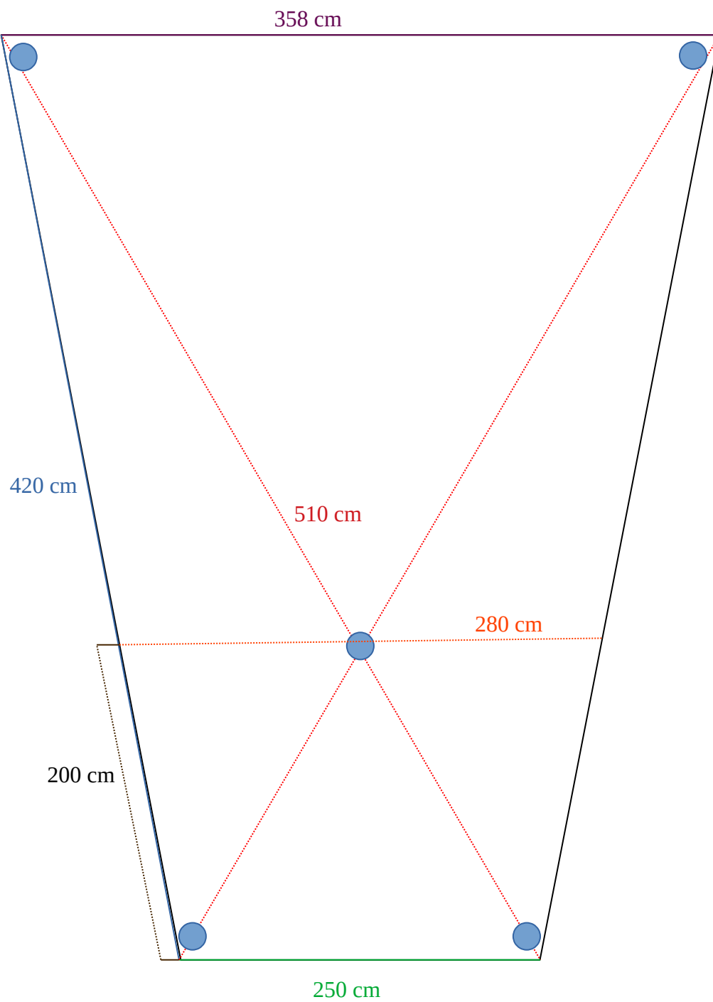
Schematyczny rysunek żagla przeciwsłonecznego z wymiarami
