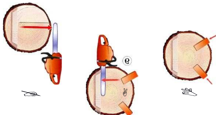
Rys.18 Technika ścinki i obalania drzewa o średnicy nie przekraczającej dwóch długości użytecznych przewodnicy.
