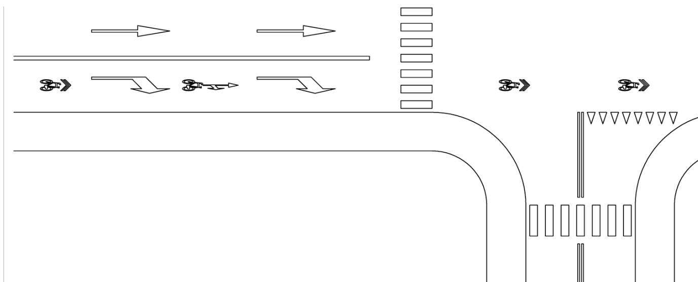
Rys. 18B. Skrzyżowanie, na którym ruch rowerów odbywa się w jezdni na zasadach ogólnych. Znak P-27 „kierunek i tor ruchu roweru” wskazuje rowerzyście miejsce na pasie ruchu ogólnodostępnego, a połączenie znaku P-23 i strzałki kierunkowej P-8f w rozmiarze „mini” umożliwia jazdę rowerem zarówno na wprost, jak i w prawo. Pozycja rowerzysty na środku pasa ruchu poprawia jego widoczność i utrudnia lub uniemożliwia niebezpieczne wyprzedzanie i zajeżdżanie mu drogi.
