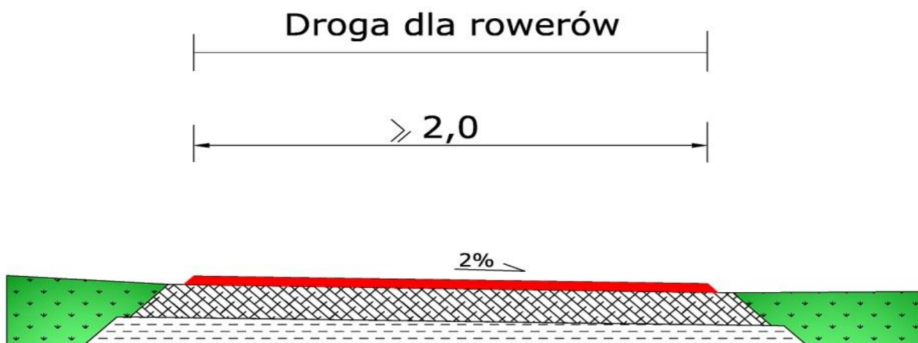
Rys. 12C. Konstrukcja drogi dla rowerów bez obrzeży (krawężników).
