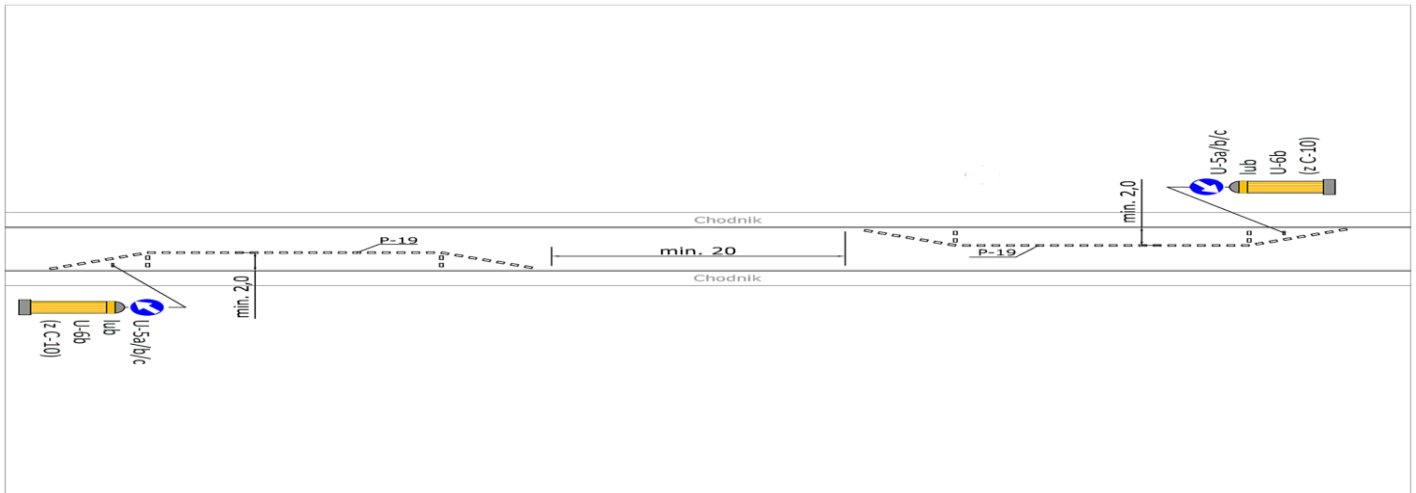
Rys. 3. Esowanie toru jazdy pojazdów przez naprzemienną lokalizację miejsc postojowych.
