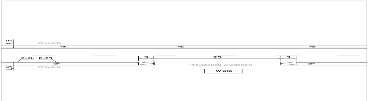
Rys. 7. Pas ruchu dla rowerów przechodzący w „przystanek wiedeński” (rodzaj przejezdnej antyzatoki).
