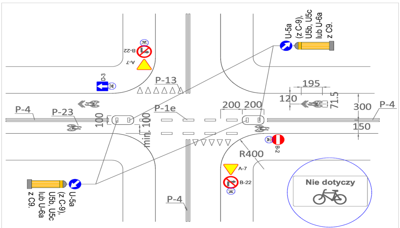
Rys. 10A. Jeśli jazda z kontrapasa jest dozwolona tylko w określonym kierunku, wówczas łącznie ze znakiem P-23 „rower” na wlocie stosuje się odpowiedni wariant strzałki kierunkowej P-8 w rozmiarze mini.
