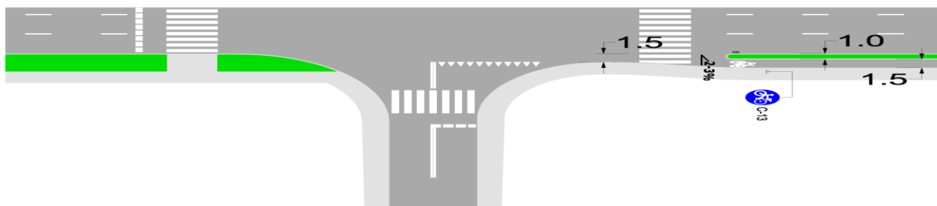
Rys. 17A. Początek jednokierunkowej drogi dla rowerów za skrzyżowaniem z poszerzeniem jezdni
