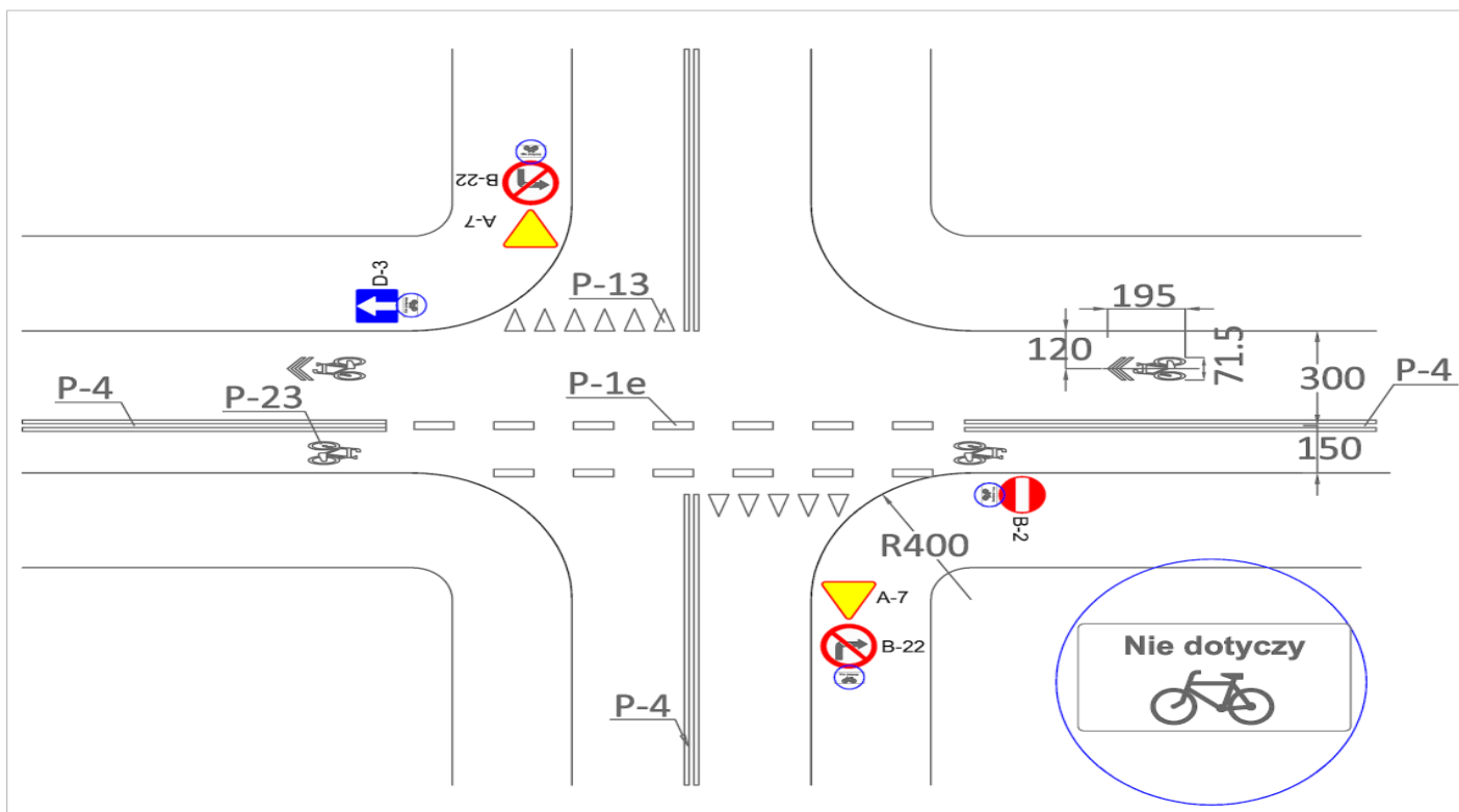
Rys. 10. Kontrapas wyznaczony w jezdni ulicy jednokierunkowej na skrzyżowaniu z ustalonym pierwszeństwem. Jeśli na skrzyżowaniu występuje duże natężenie pojazdów samochodowych na relacji skrętnej z drogi z pierwszeństwem, na wlocie umieszcza się wyspę dzielącą ze słupkiem U-5a/b/c (patrz rys. 10B).
