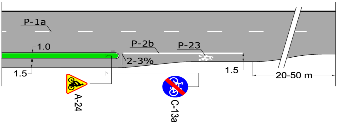
Rys. 17C. Koniec jednokierunkowej drogi dla rowerów
