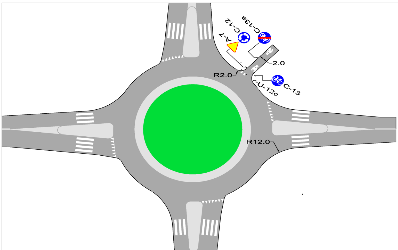
Rys. 23A. Dwukierunkowa droga dla rowerów jako samodzielny wlot małego ronda.
