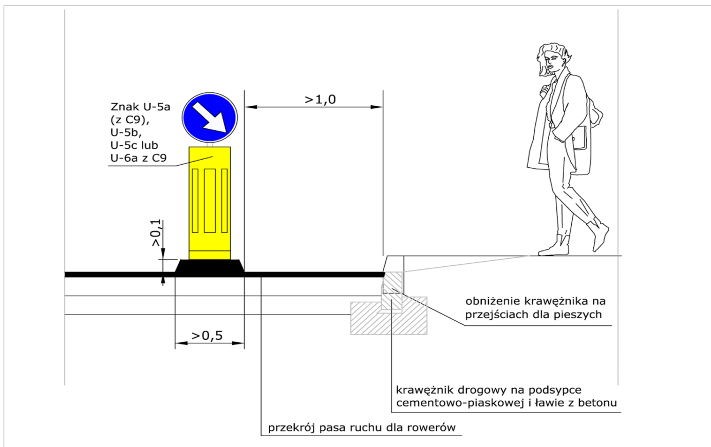
Rys. 11. Wyspa dzieląca ze słupkiem przeszkodowym U-5a/b/c (lub tablicą U-6a) oddzielająca pas ruchu dla rowerów (kontrapas) od pozostałej części jezdni. Widoczne dopuszczalne wyjątkowo zwężenie pasa ruchu dla rowerów do 1,0 m w poziomie niwelety.
