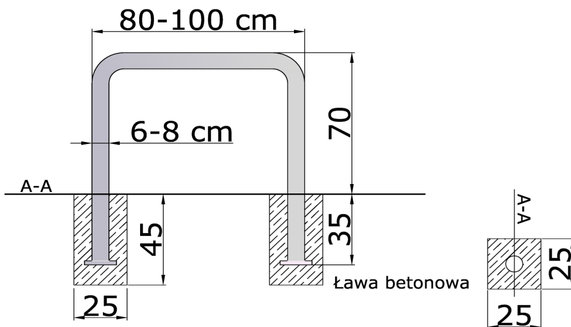
Rys. 25A. Przykładowy stojak rowerowy „odwrócone U”.
