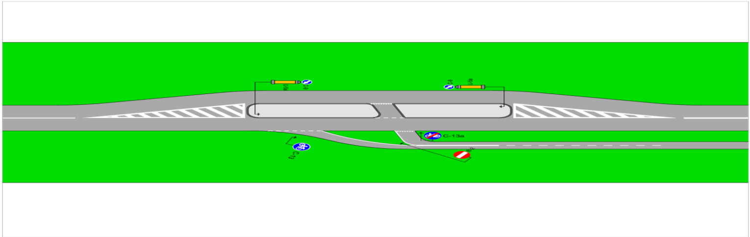
Rys. 17D. Zakończenie dwukierunkowej drogi dla rowerów z wprowadzeniem ruchu rowerów w jezdnię na podporządkowaniu przez azyl wytworzony przez wyspę dzielącą między pasami ruchu. Zjazd z jezdni na drogę dla rowerów odbywa się z zachowaniem parametrów geometrycznych określonych na rysunku 17B.
