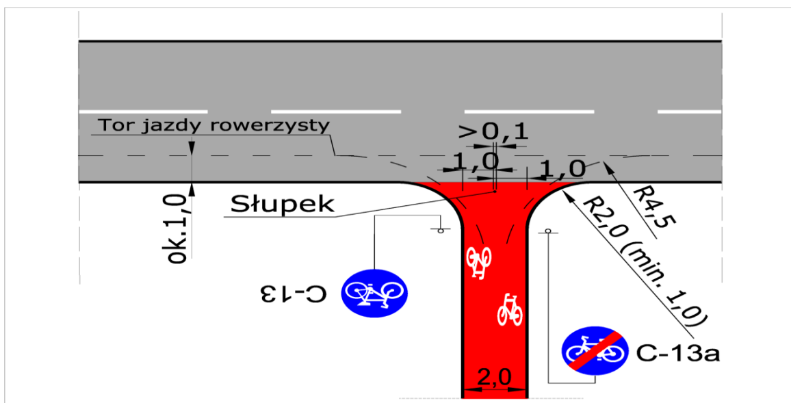
Rys. 17E. Wlot dwukierunkowej drogi dla rowerów biegnącej prostopadłe do jezdni ogólnodostępnej z dopuszczonym ruchem rowerów. Aby ułatwić wjazd na drogę dla rowerów i opuszczenie jej zastosowano wyokrąglenia styku krawędzi jezdni ogólnodostępnej i drogi dla rowerów. Na rysunku przedstawiono orientacyjny tor jazdy rowerzystów i położenie słupków blokujących U-12c.
