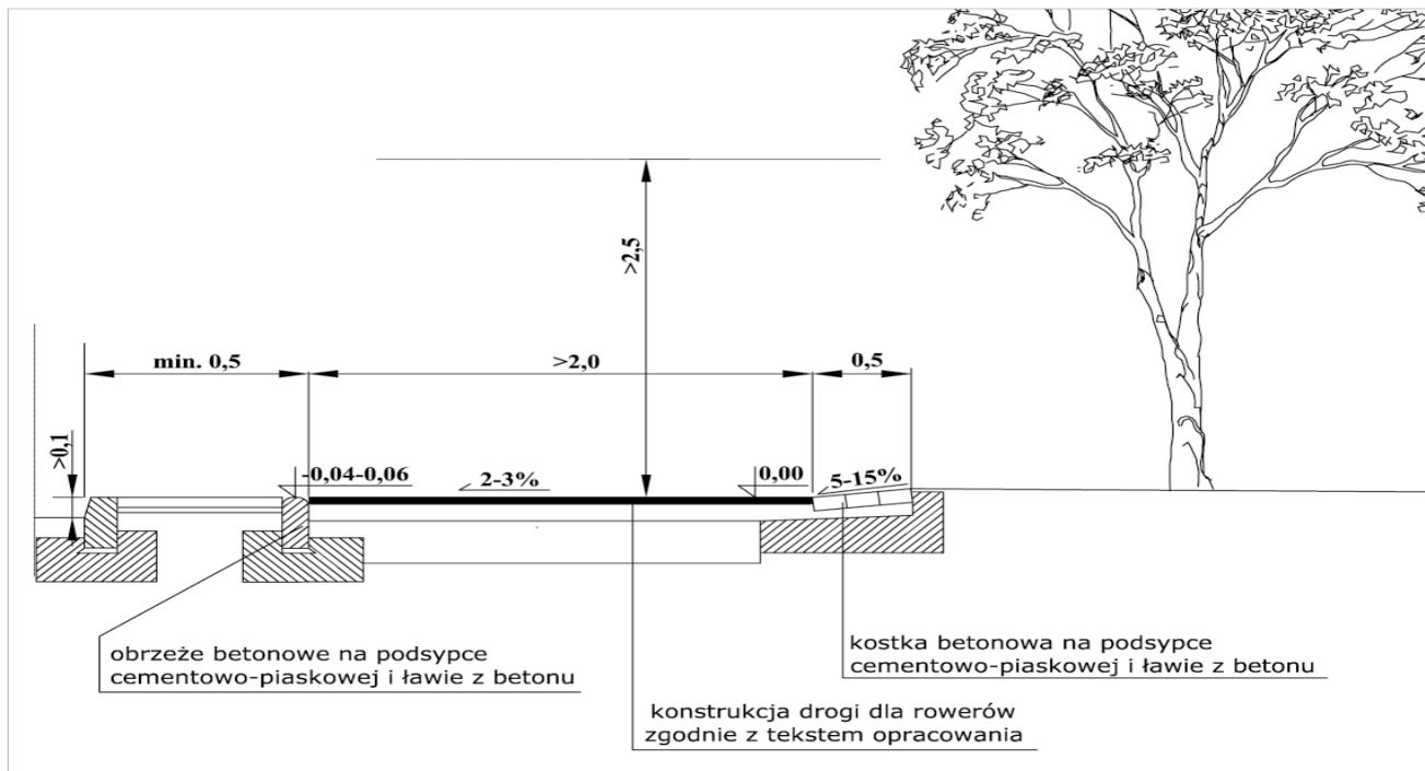
Rys. 12A. Przekrój poprzeczny dwukierunkowej drogi dla rowerów o nawierzchni bitumicznej, zamkniętej obrzeżem i opaską z kostki brukowej oddzielającą ją od chodnika (nie przedstawiony na rysunku).
