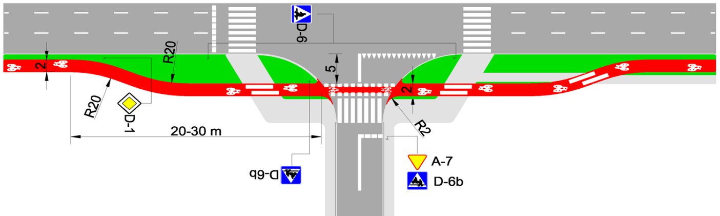
Rys. 21. Poprawny przebieg drogi dla rowerów w rejonie skrzyżowania: duże promienie łuków w dużej odległości od przejazdu dla rowerzystów. Zwracają uwagę wyokrąglenia na styku drogi dla rowerów i jezdni ogólnodostępnej.
