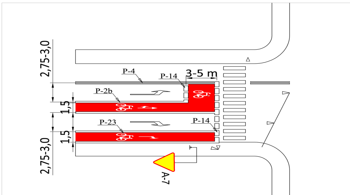
Rys. 20A. Śluza typu 1 (klasyczna). Patrz też rys. 19A i 19B.
