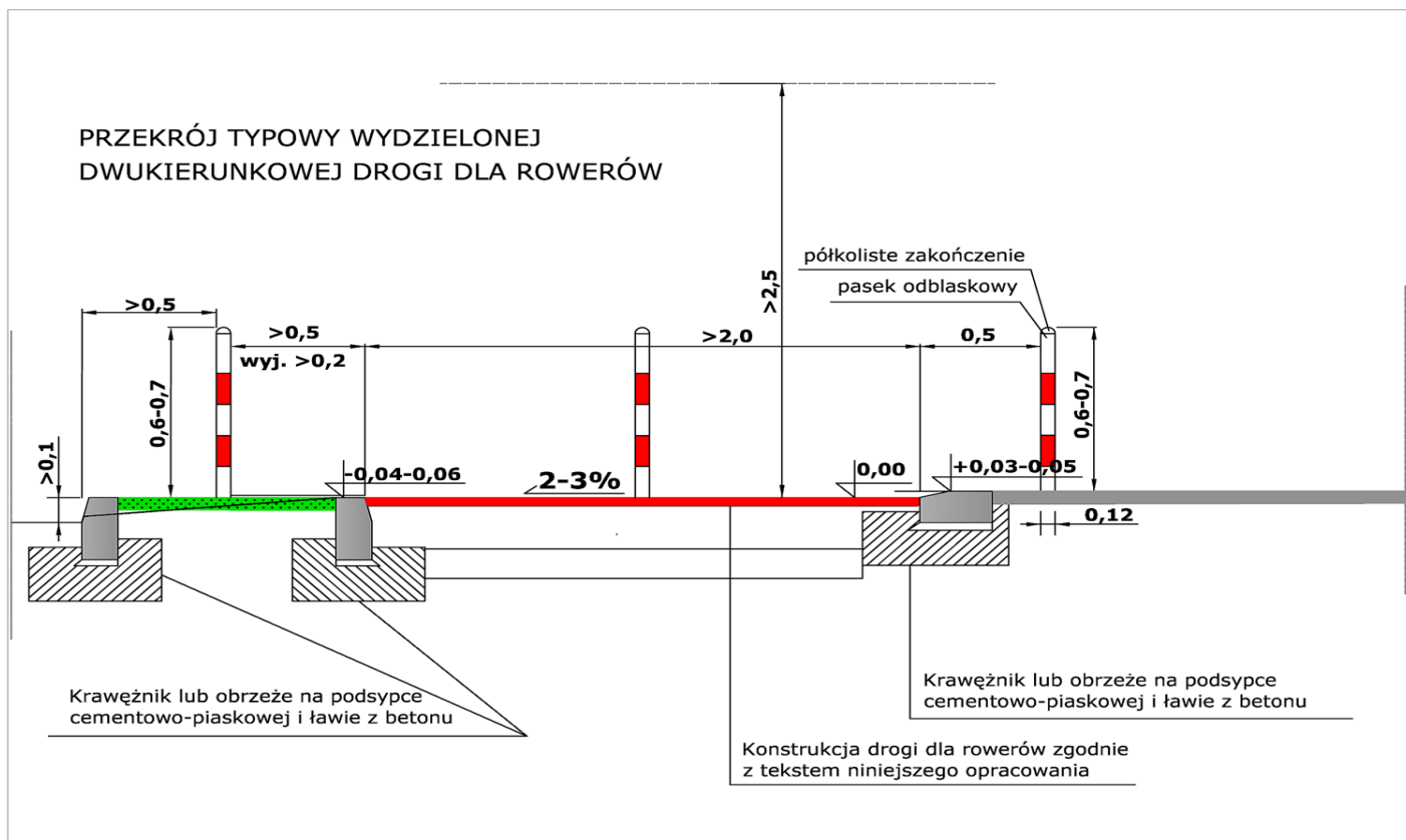
Rys. 13. Zasady lokalizacji słupków blokujących U-12c w przekroju dwukierunkowej drogi dla rowerów. Jeden słupek musi znajdować się symetrycznie w osi drogi dla rowerów. Od jezdni dodatkowo drogę dla rowerów może oddzielać bariera ochronna U-14a. W przekroju zaznaczono dodatkowo skos zjazdu indywidualnego (słupki blokujące stosuje się m. in. w rejonie zjazdów, którymi samochody mogą nielegalnie wjeżdżać na drogę dla rowerów).
