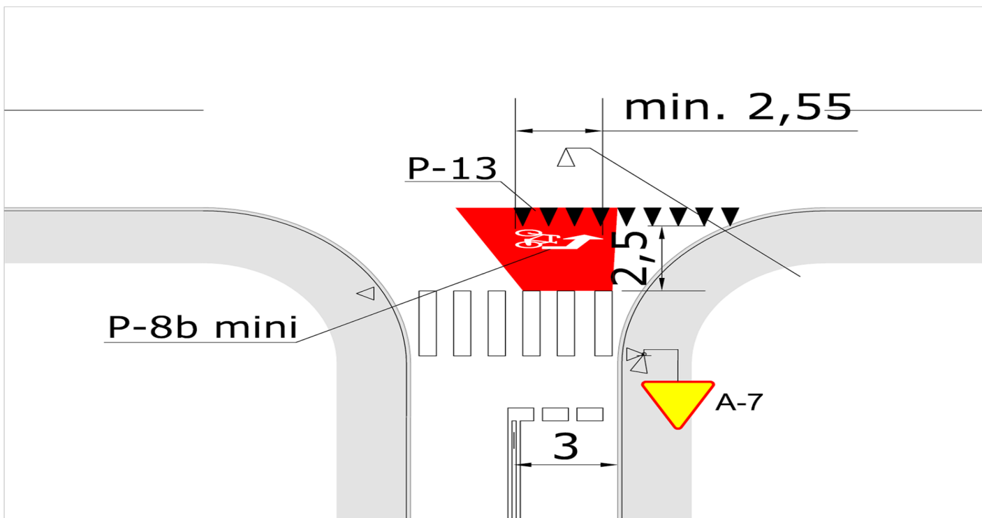
Rys. 20B. Śluza typu 2 zlokalizowana na wlocie podporządkowanym, wloty z pierwszeństwem bez pasa ruchu dla rowerów, przejście dla pieszych przez wlot podporządkowany i sygnalizacja świetlna. Czerwona nawierzchnia śluzy nie jest zwymiarowana (nie stanowi znaku drogowego).
