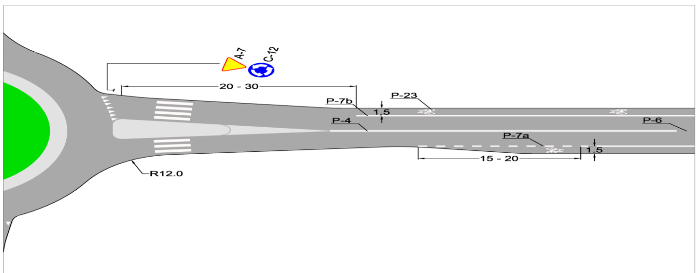
Rys. 18A. Małe rondo z wlotem przed którym pas ruchu dla rowerów został obcięty.
