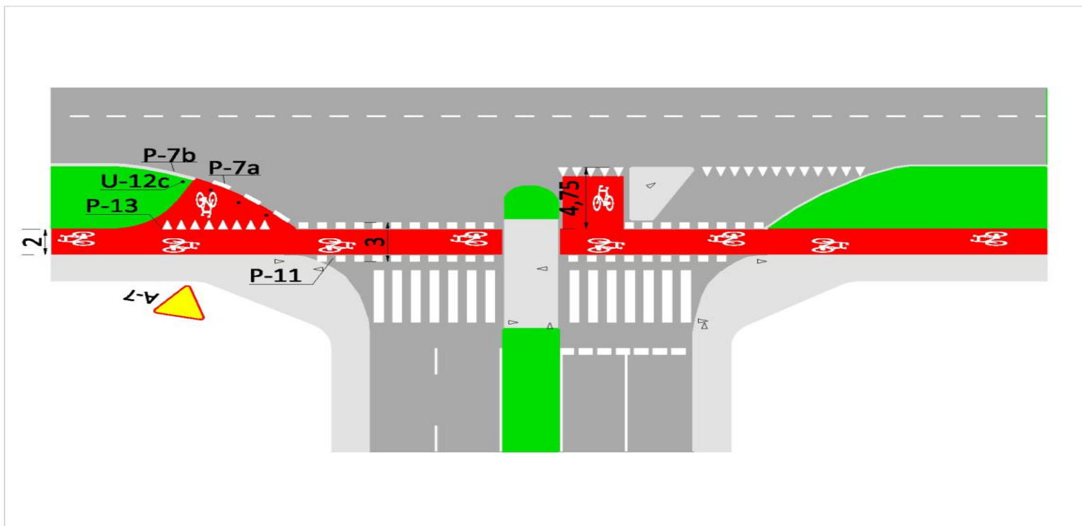
Rys. 20D. Droga dla rowerów i przejazd dla rowerzystów ze śluzami do skrętu w stronę skrzyżowania (typu 3, pośrodku) i do skrętu na drodze dla rowerów (typu 4, w lewym narożniku) umożliwiającymi bezpieczne pokonanie skrzyżowania na relacjach nie obsługiwanych drogami dla rowerów. Część oznakowania pionowego pominięto.
