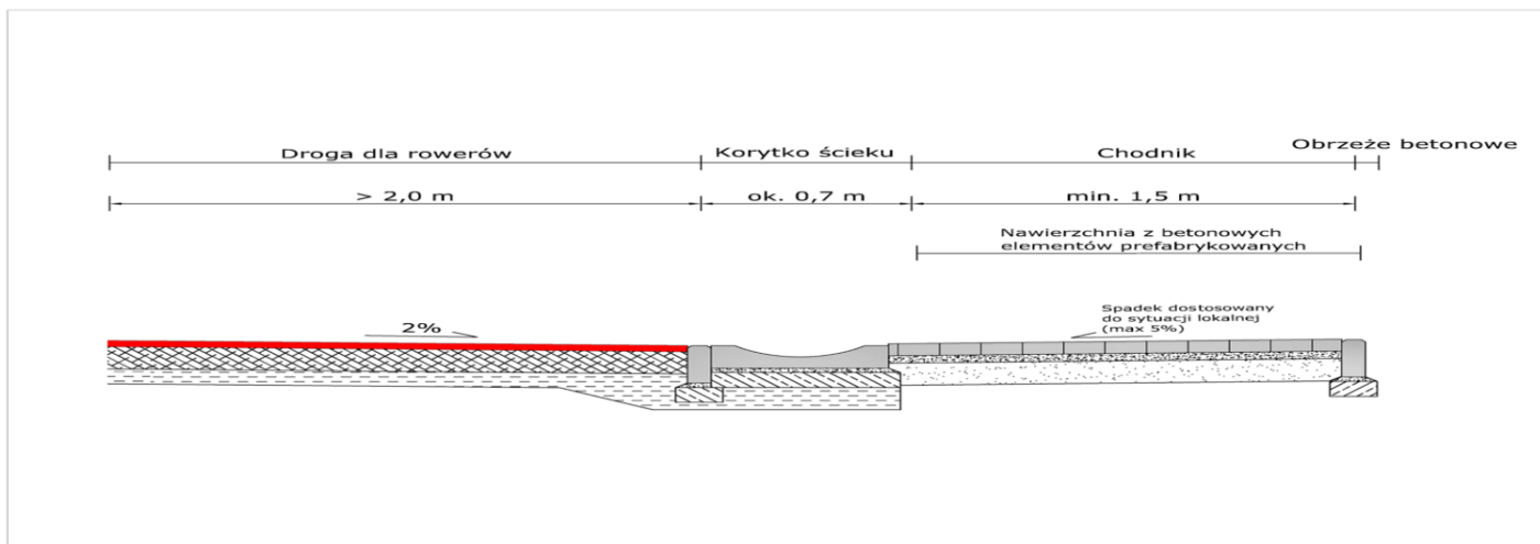
Rys. 12D. Przykład konstrukcji dwukierunkowej drogi dla rowerów oddzielonej od chodnika prefabrykowanym otwartym ściekiem korytkowym o przekroju wycinka koła.
