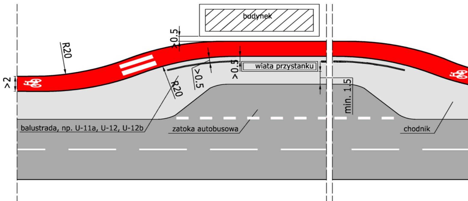
Rys. 16. Przykładowy przebieg drogi dla rowerów w rejonie przystanku autobusowego
